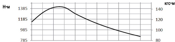
Крутящий момент
