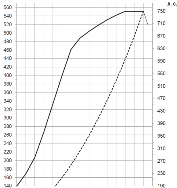
Мощность кВт
