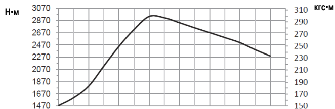
Крутящий момент
