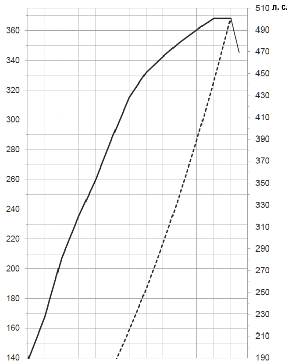
Крутящий момент
